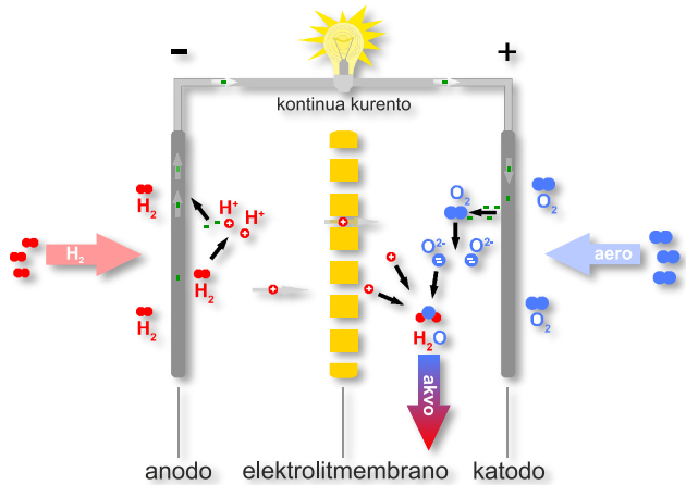
Funkcprincipo fuelpila
