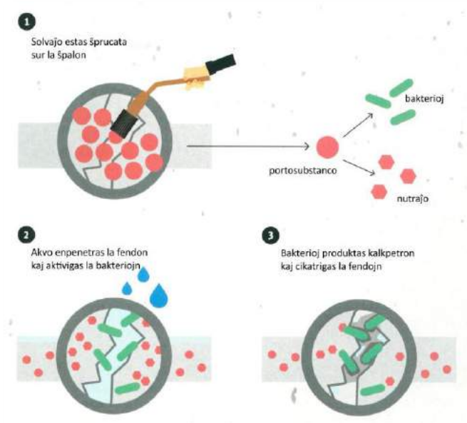
Traktado de ŝirfendita betonŝpalo (skemo: DB Welt)
